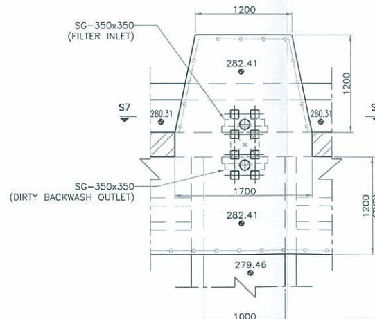
DETAIL-E SCALE 1:30
