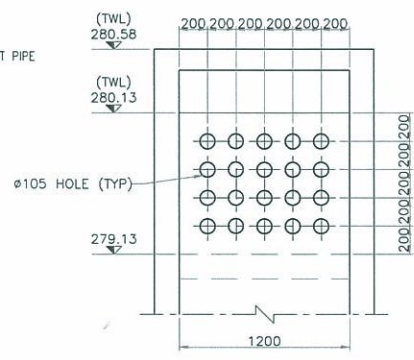
DETAIL-D SCALE 1:25
